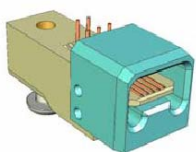
USB plug mini Type B with center unit
